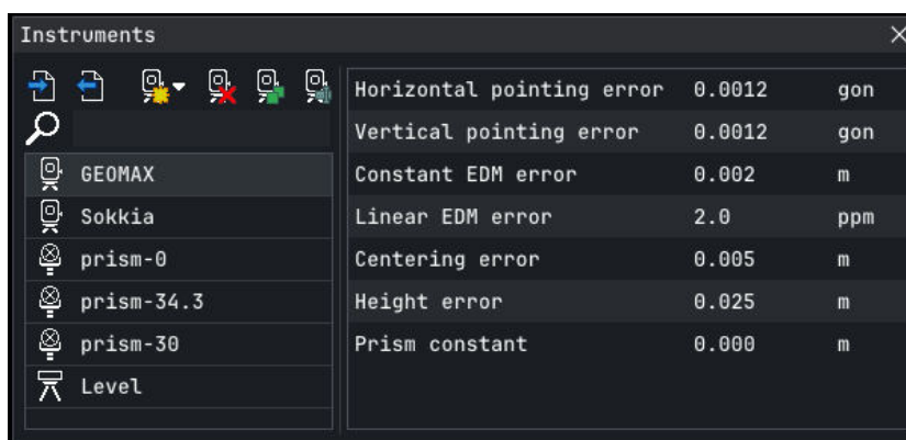
Фиг.1. Параметри на точността за тотална станция „GEOMAX“
