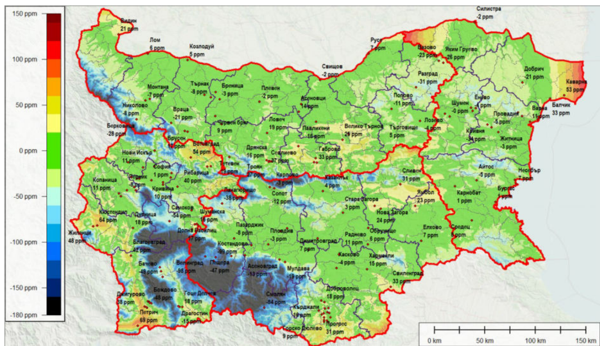
Фиг. 6. Комбинирана карта на деформациите при Вариант 2 (четири LDP зони)
