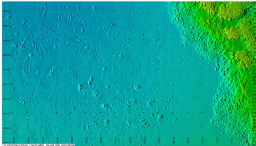
Фиг.6. Свръх детайлен теренен модел измерен с многолъчев ехолот с разделителна способност 20x20 см, дълбочина до 20 метра. Моделът е в района на потъналата вкаменена гора до гр. Созопол. Отчетливо се идентифицират останките от дървесни пънове, полегнали дървета и други обекти по дъното.
